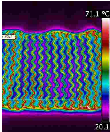
Wärmebild beheizbares Verbundgewirke für Sitzflächen, entwickelt am STFI Chemnitz, (c) STFI
